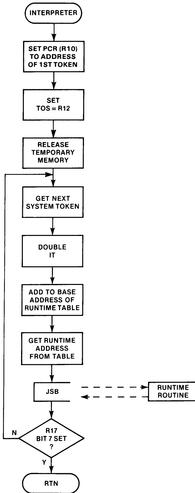
INTERPRETER LOOP
