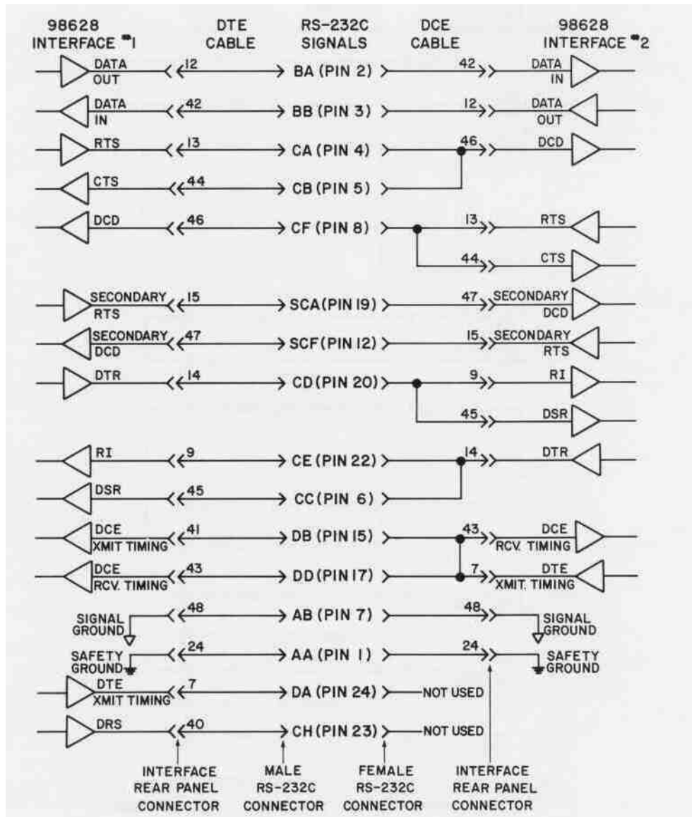
DTE/DCE Interface Cable Wiring
