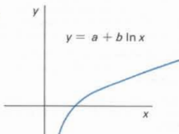
Logarithmische Regression Code = 2
